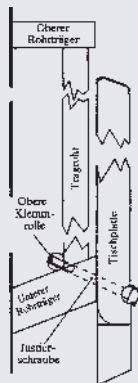
Montageskizze 2 - Tischplatte eingeklappt
