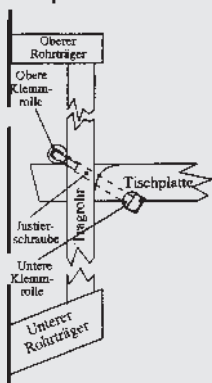
Montageskizze 1 - Tischplatte in Funktion
